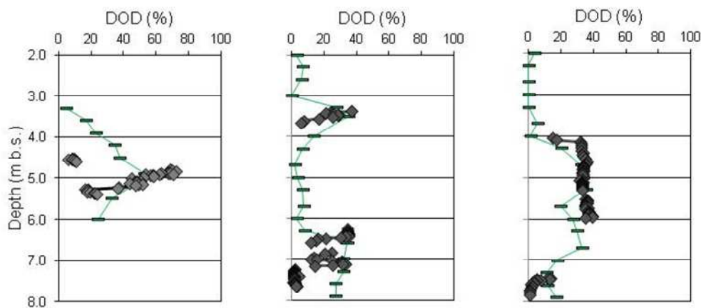
Figur 9b: Sammenligning af DOD beregnet fra MIP GC data og fra kerneprøve data for C1, C2 og C3 (fra venstre mod højre).
