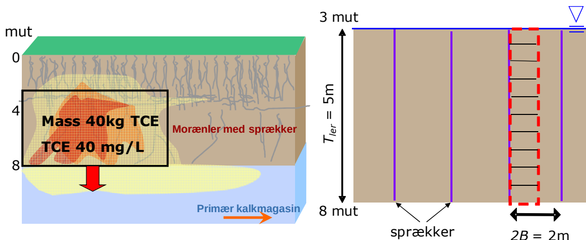
Figur 24: Den konceptuelle model brugt til modelleringen af Gl. Kongevej. TCE koncentrationen til tiden 0 (før oprensningen er opstartet) er antaget at være homogen i kildeområdet. Simplifikation af modellen er vist til højre: sprækkerne (lilla linier) er antaget at findes med samme afstand og at være gennemtrængelige hele vejen. Model domænet er vist (rød stiplede kasse). Injektionsdybderne er vist som sorte horisontale linier med 25 cm afstand.
