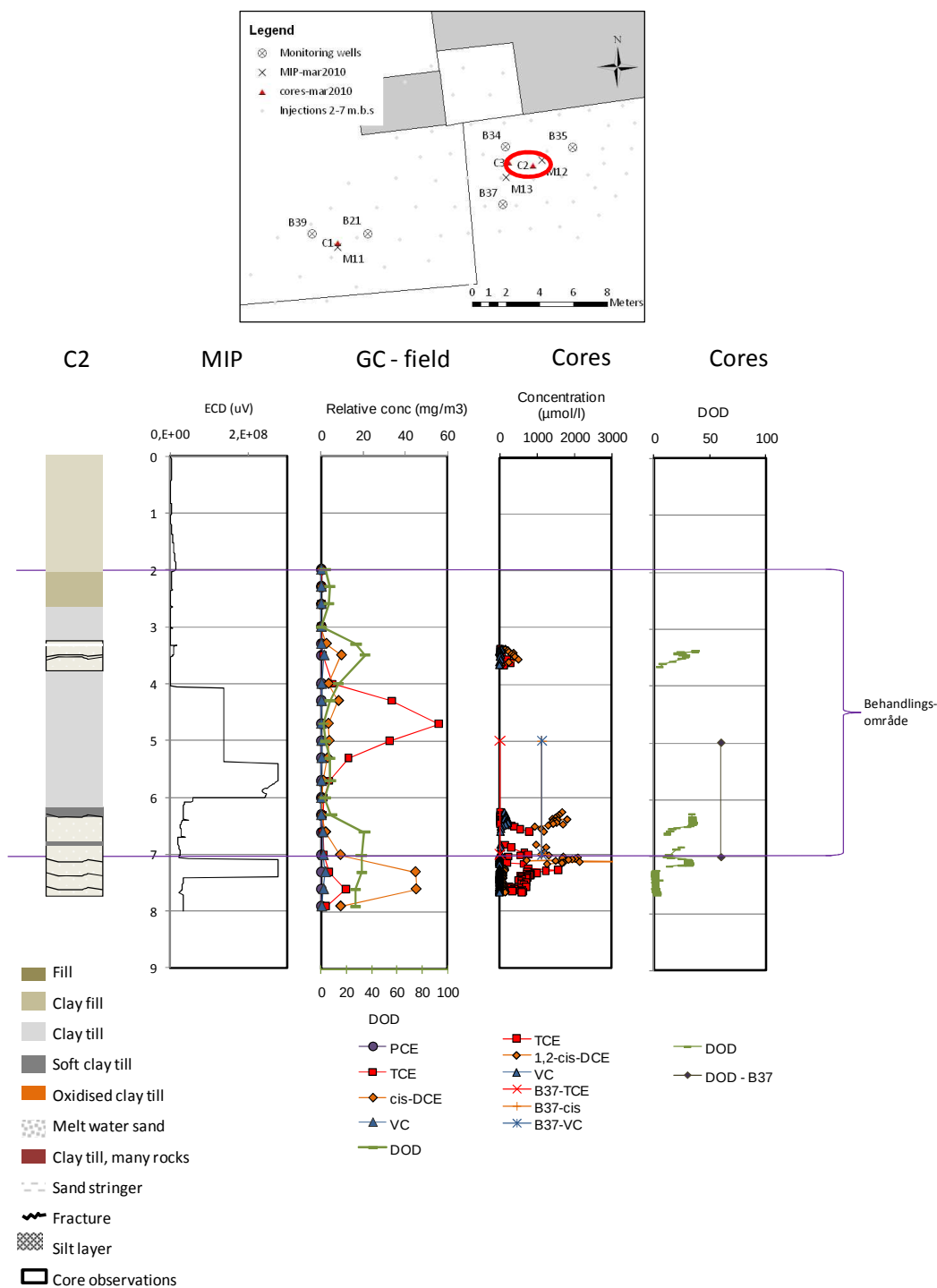
Figur 10: Den geologiske beskrivelse af C2 (kildeområdet) baseret på borningsobservationer og kernebeskrivelser. Endvidere ses resultatet af ECD ved MIP, den relative koncentration af chlorerede ethener målt på felt GC under MIP, koncentrationen af chlorerede ethener målt i kerneprøverne og i grundvand fra nærliggende boring, samt den beregnede DOD beregnet ud fra målte koncentrationer i kerneprøverne og grundvandet.
