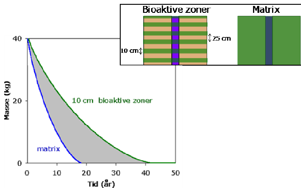
Figur 25: To model scenarier er vist. Scenarie et: bioaktive zoner med en bredde på 5 cm på hver side af injektionsdybden. Scenarie to: Nedbrydning i hele matricen. Modelresultaterne for massefjernelsen er vist nederst til venstre. Resultaterne fra modelleringen viser at massefjernelsen (100%) tager mellem 20 og 40 år.
